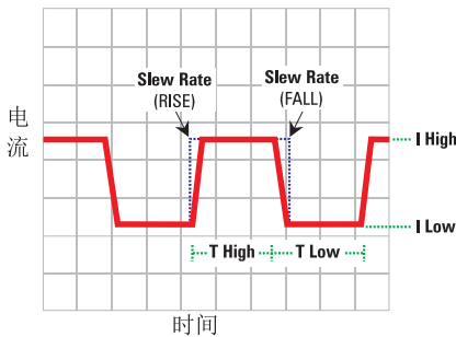
图4 - 直流型号动态模式
