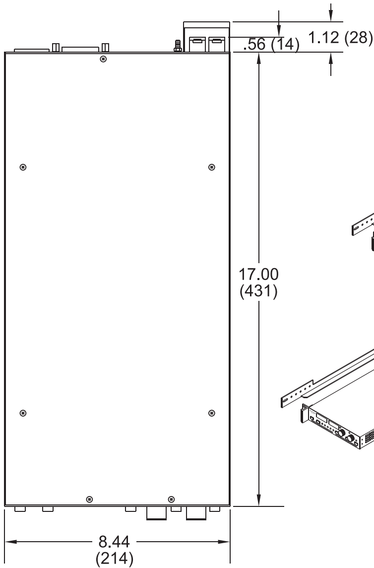
顶视图
