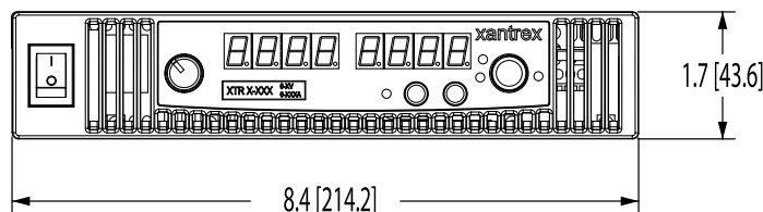
正视图
