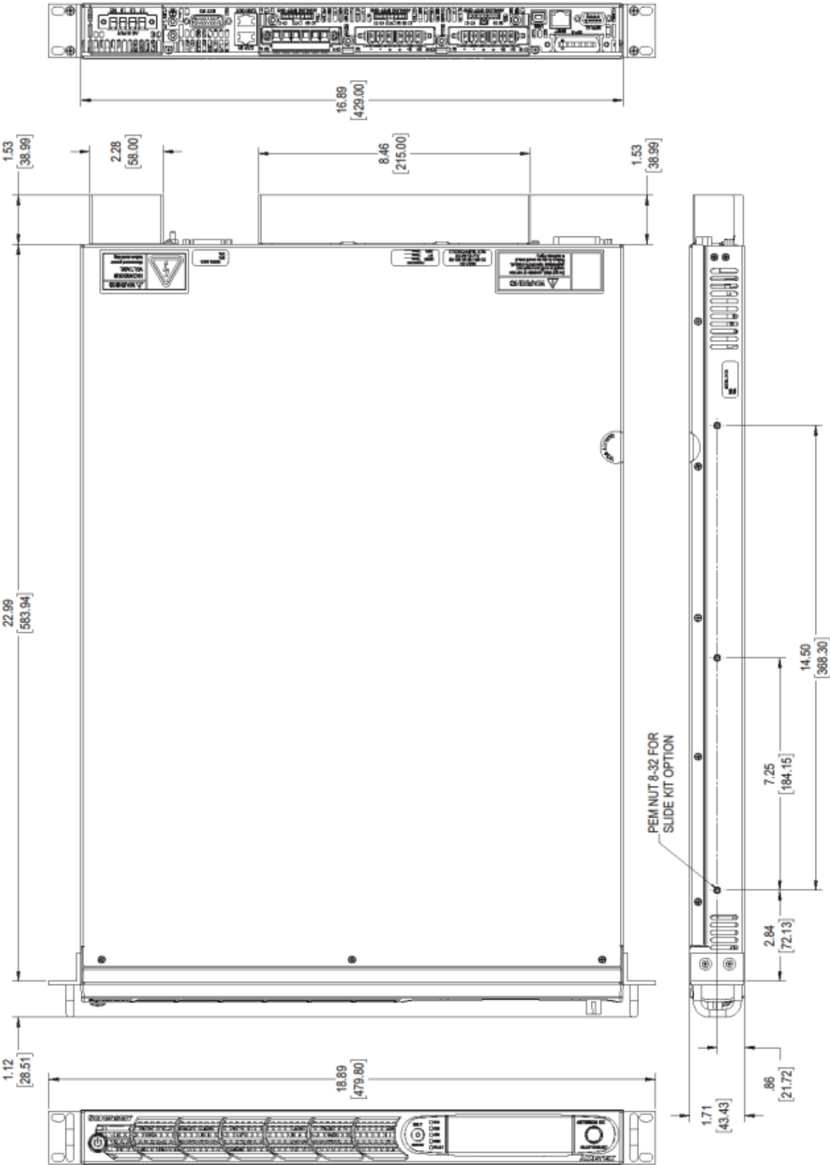
机箱尺寸图 (1U)
