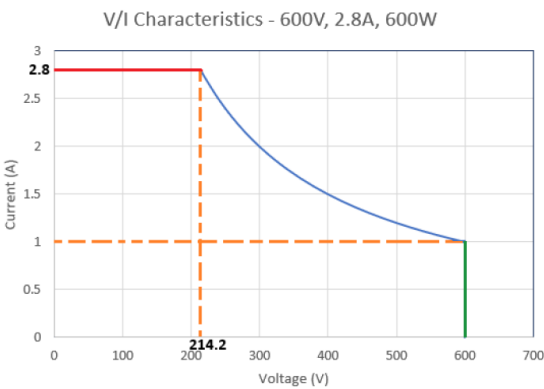
ASA 系列 600W-600V-2.8A 型号 I-V 输出曲线
