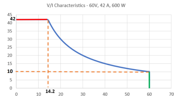
ASA 系列 600W-60V-42A 型号 I-V 输出曲线
