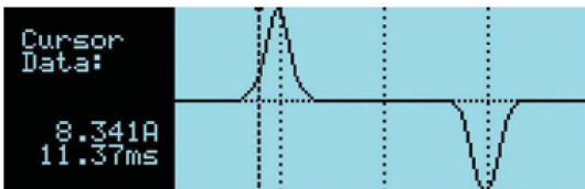
电压波形获取(前面板显示)
