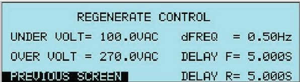
-SNK模式界面
