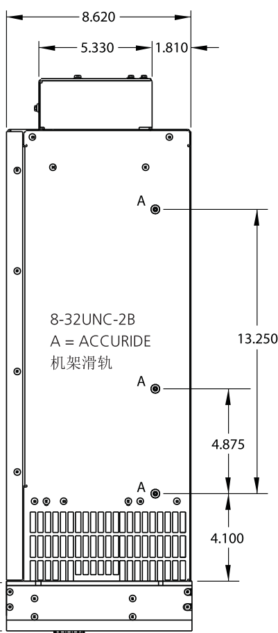
侧视图
